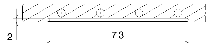
VISTA CORTE SECCIÓN A-A ESCALA 1:1
