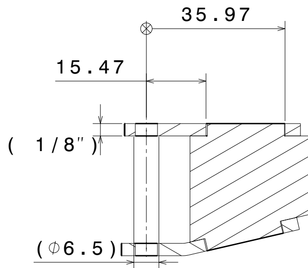
VISTA CORTE SECCIÓN B-B
