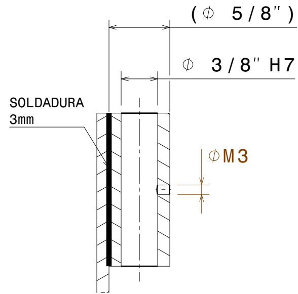
VISTA CORTE SECCIÓN A-A
