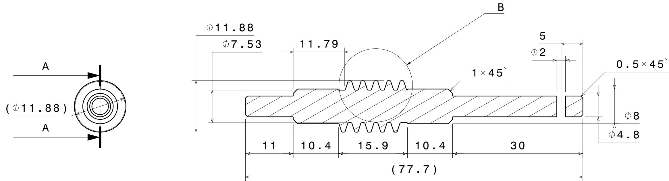
SECCION A-A
