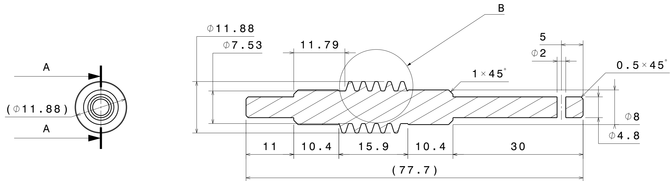
SECCION A-A
