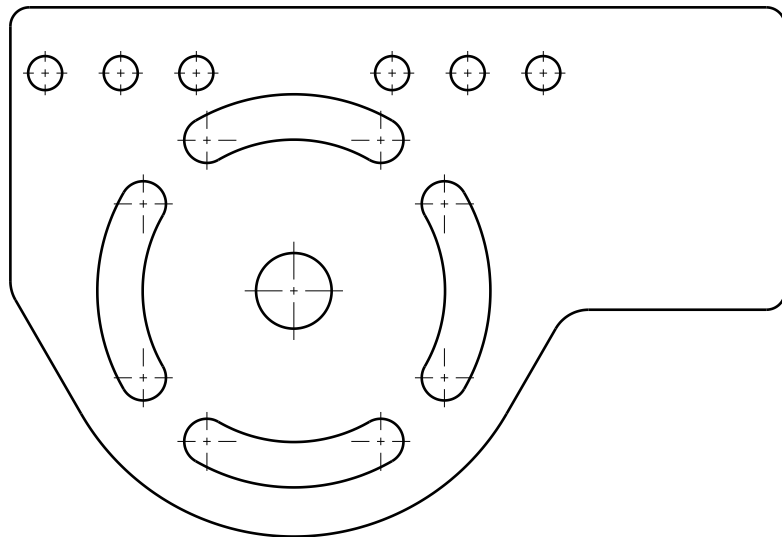
PLANTILLA DE CORTE POR LASER PIEZA: 1.1 ESPESOR: 1/8" CANTIDAD: 2 PIEZAS MATERIAL: PLACA ASTM A-36
