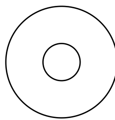
PLANTILLA DE CORTE POR LASER PIEZA: 1.2 ESPESOR: 3/16" CANTIDAD: 4 PIEZAS MATERIAL: PLACA ASTM A-36
