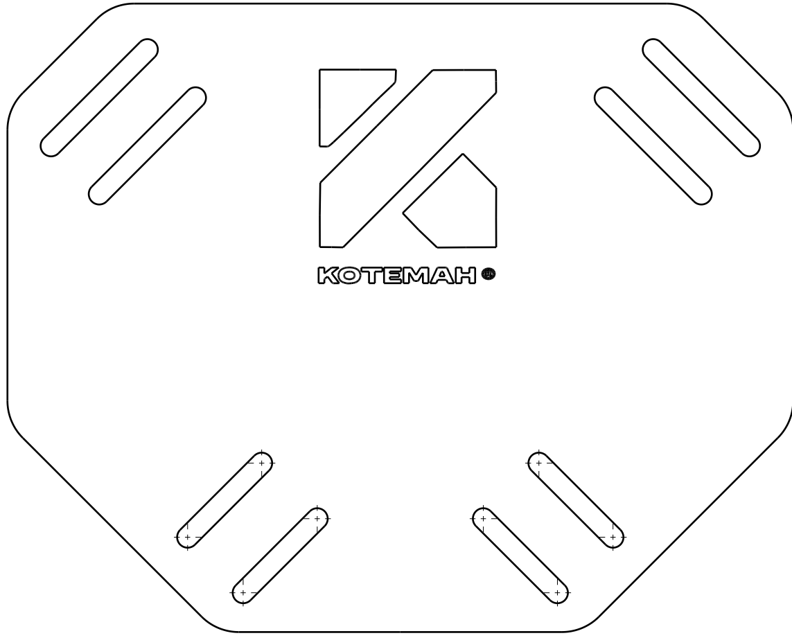
PLANTILLA DE CORTE POR LASER PIEZA: 1.1 ESPESOR: 1/8" CANTIDAD: 1 PIEZA MATERIAL: PLACA ASTM A-36
