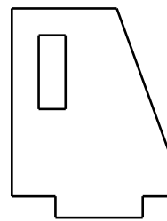
PLANTILLA DE CORTE POR LASER PIEZA: 4.2 ESPESOR: 1/8" CANTIDAD: 2 PIEZAS MATERIAL: PLACA ASTM A-36
