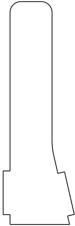
PLANTILLA DE CORTE POR LASER PIEZA: 2.1 ESPESOR: 1/8" CANTIDAD: 2 PIEZAS MATERIAL: PLACA ASTM A-36
