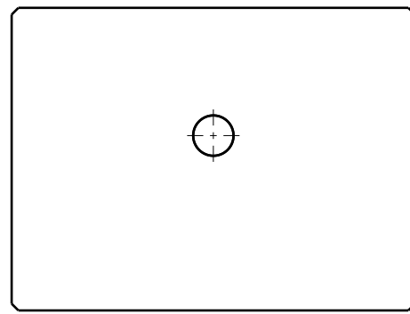
PLANTILLA DE CORTE POR LASER PIEZA: 9 ESPESOR: 1/4" CANTIDAD: 2 PIEZAS MATERIAL: PLACA ASTM A-36
