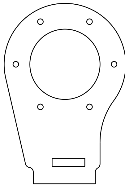
PLANTILLA DE CORTE POR LASER PIEZA: 5.1 ESPESOR: 1/8" CANTIDAD: 2 PIEZAS MATERIAL: PLACA ASTM A-36
