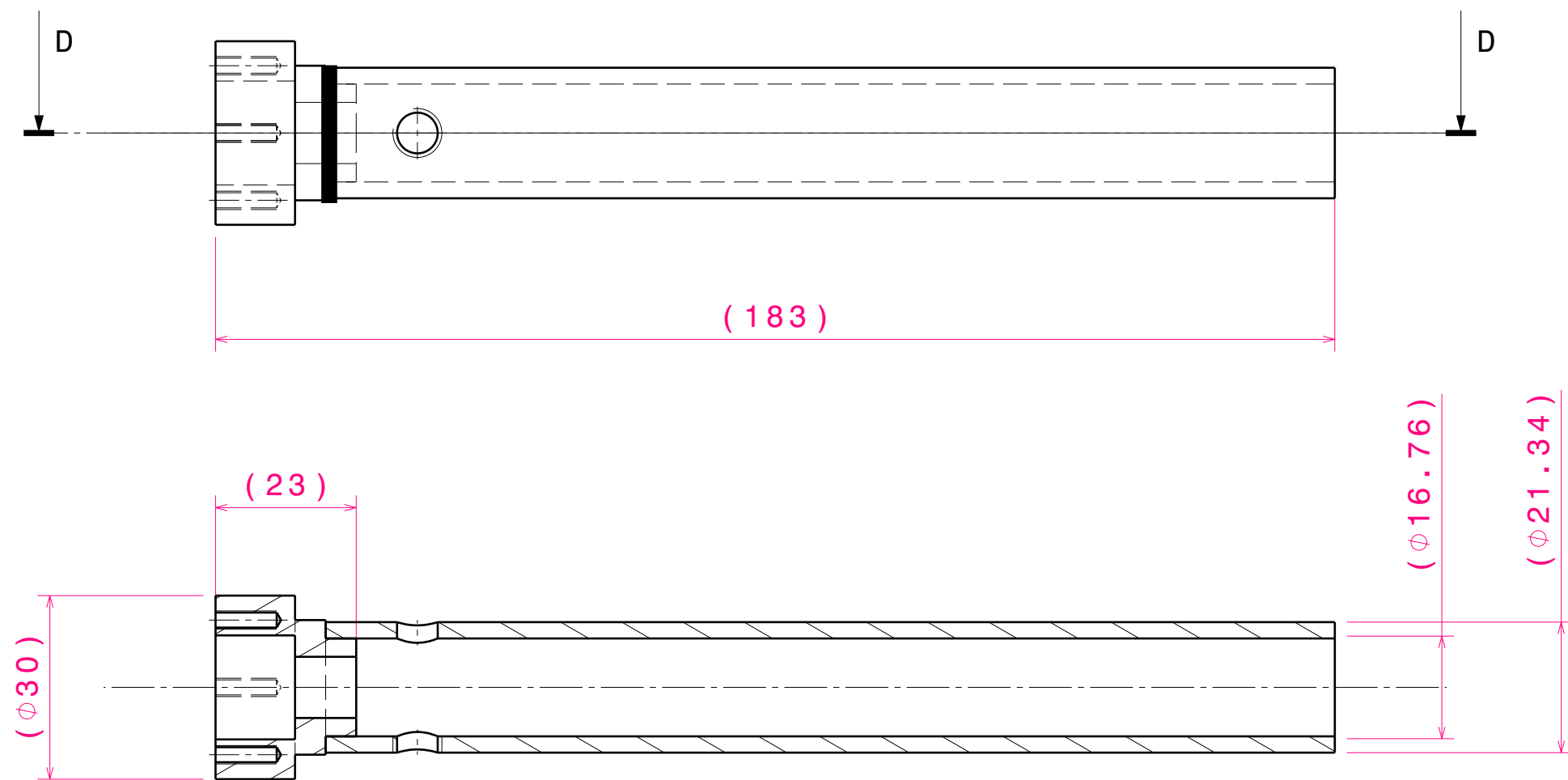
CORTE D-D
