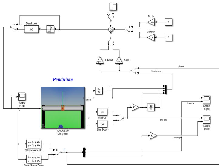
Obrázek 17: Zapojení stavové zpětné vazby s předfiltrem
