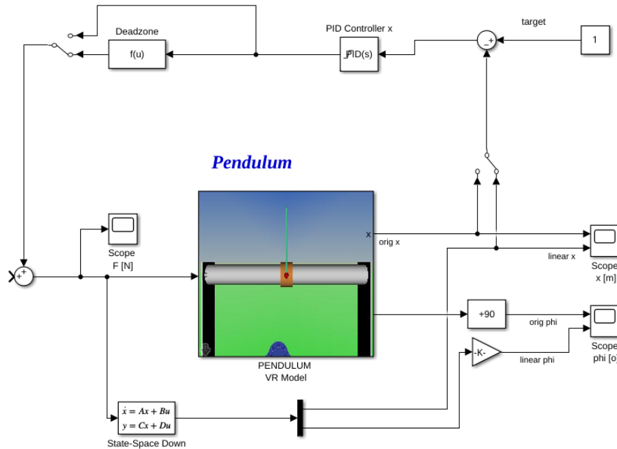
Obrázek 3: Simulink schéma pro regulátor polohy vozíku
