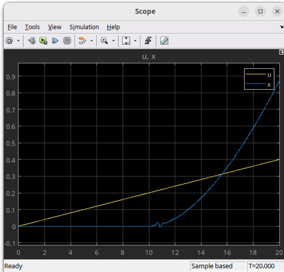
Obrázek 2: Zjišťování deadzone
