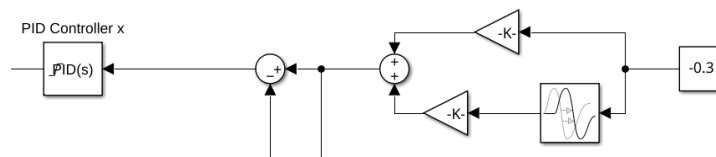
Obrázek 14: Implementace posicastu
