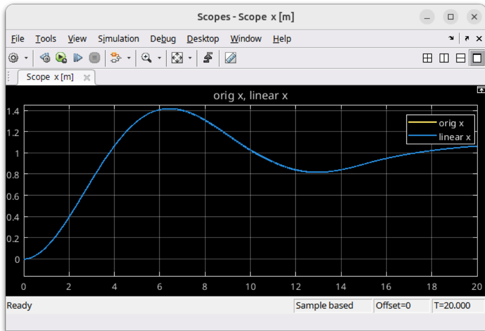
Obrázek 12: Překmit P regulátoru
