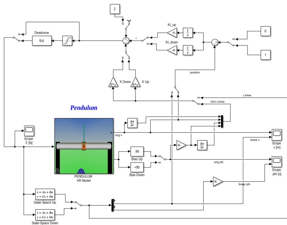
Obrázek 37: Zapojení stavové zpětné vazby s integrálním řešením v Simulinku
