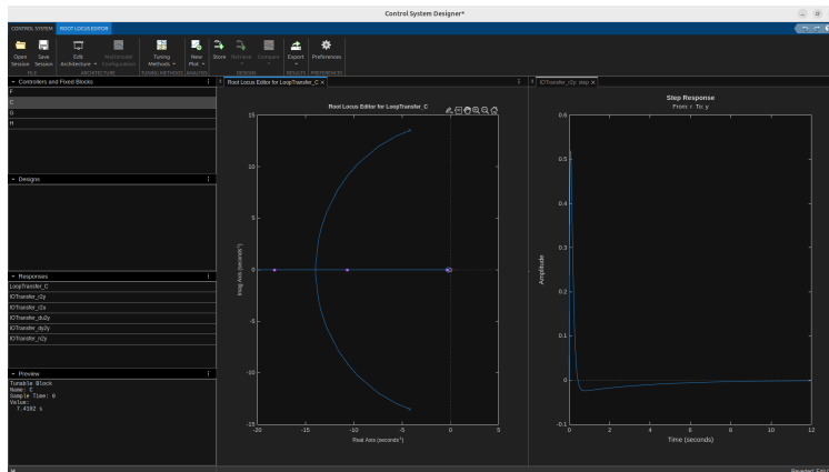
Obrázek 10: Hledání paramterů D regulátoru pomocí rltool
