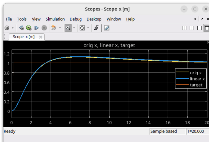
Obrázek 14: Poloha vozíku s poisicastem
