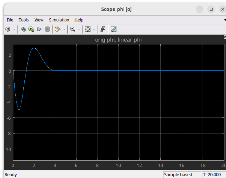
Obrázek 12: Kmitání s regulátorem
