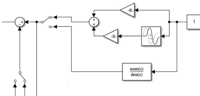
Obrázek 13: Implementace posicastu
