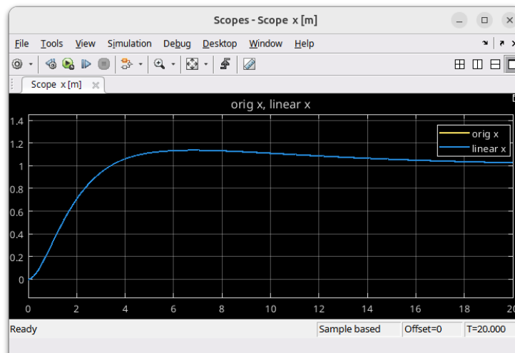
Obrázek 8: Regulace vozíku na polohu x = 1
