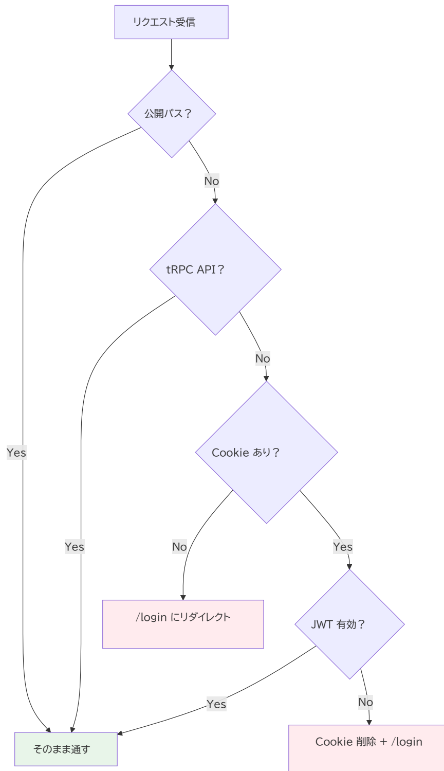
図6: コラム: middleware は「どこ」で動くのか
