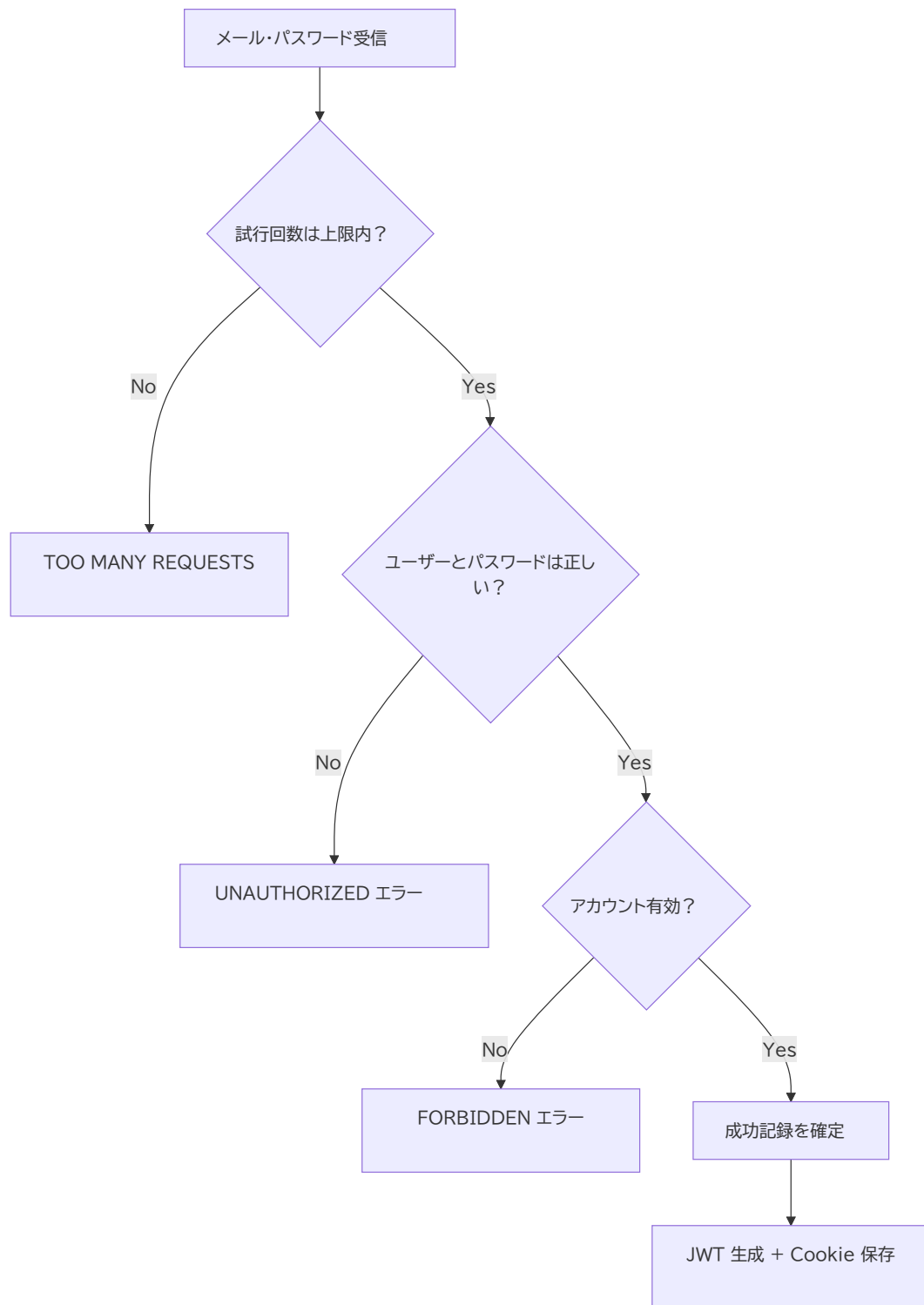
図3: 3-2. エラーハンドラーとログイン処理
