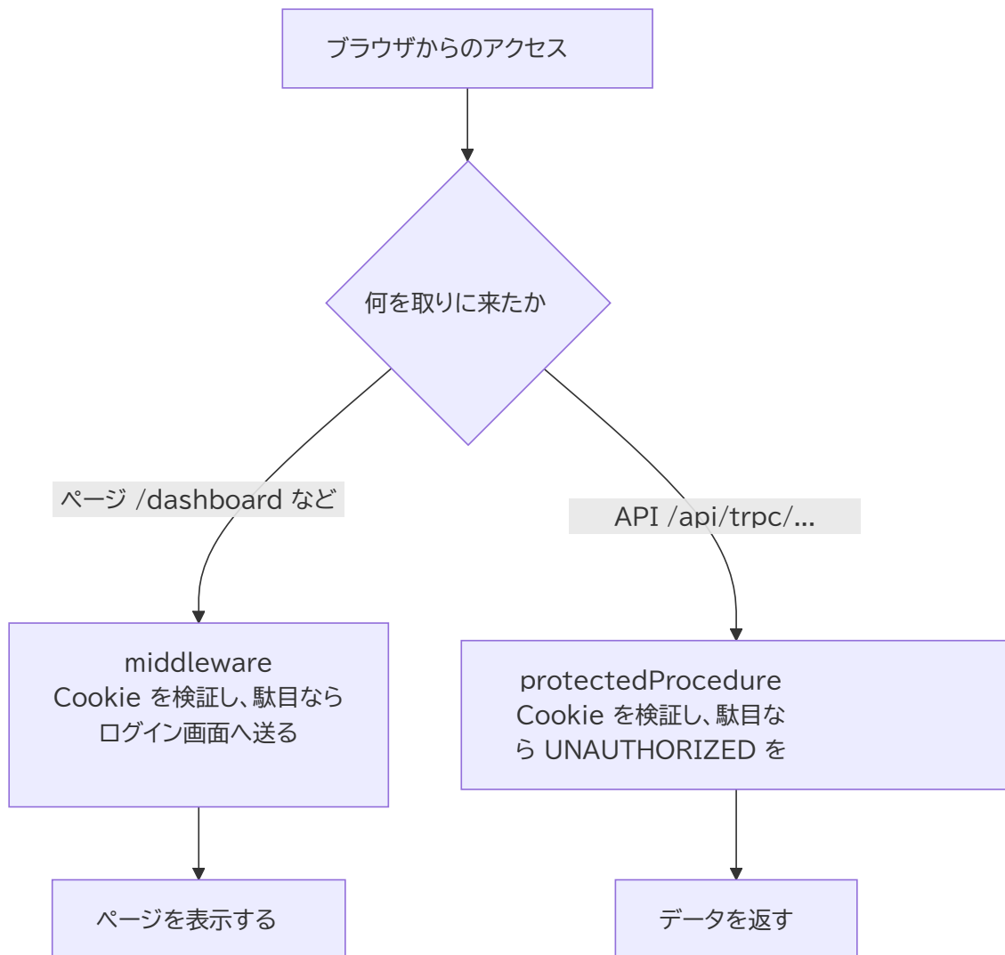
図5: Step 5: middleware.ts を作る
