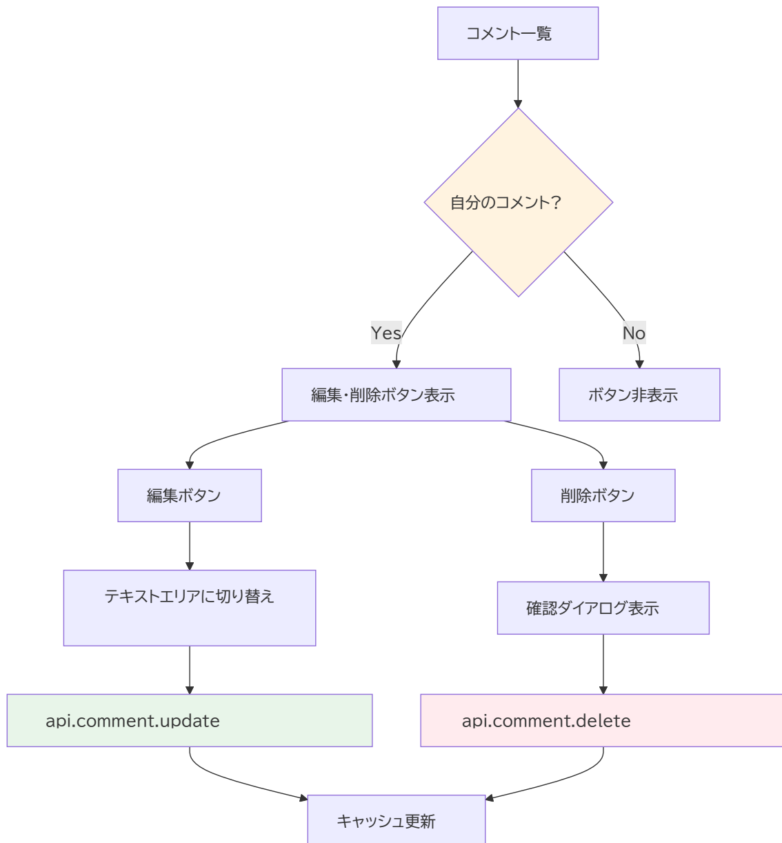
図 2: 編集・削除のフロー
