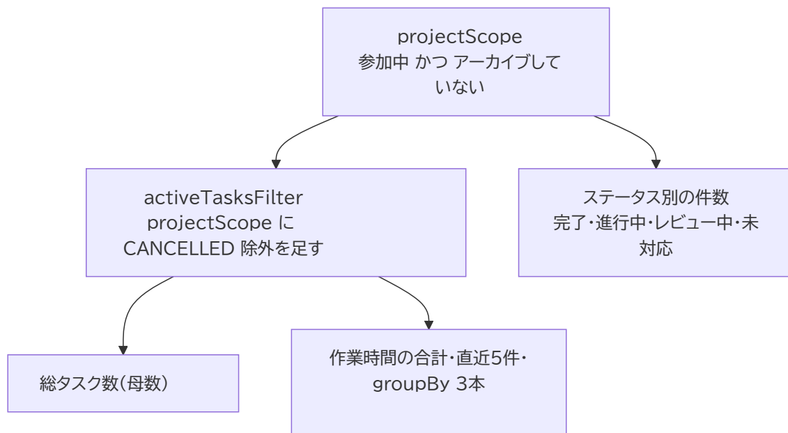
図3: 0-3. 集計の土台となる条件を作る
