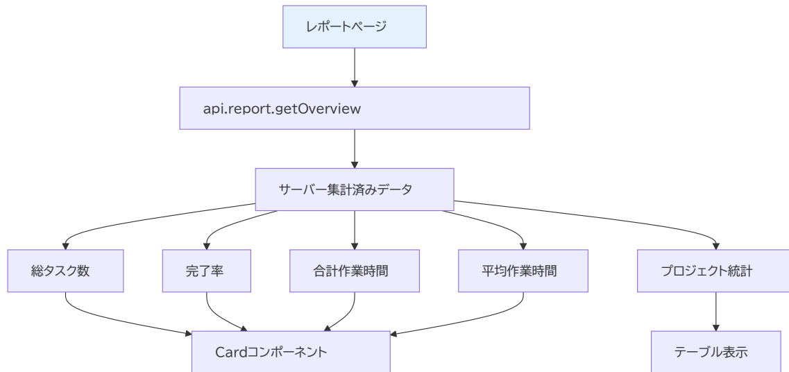
図 2: レポートページのデータフロー
