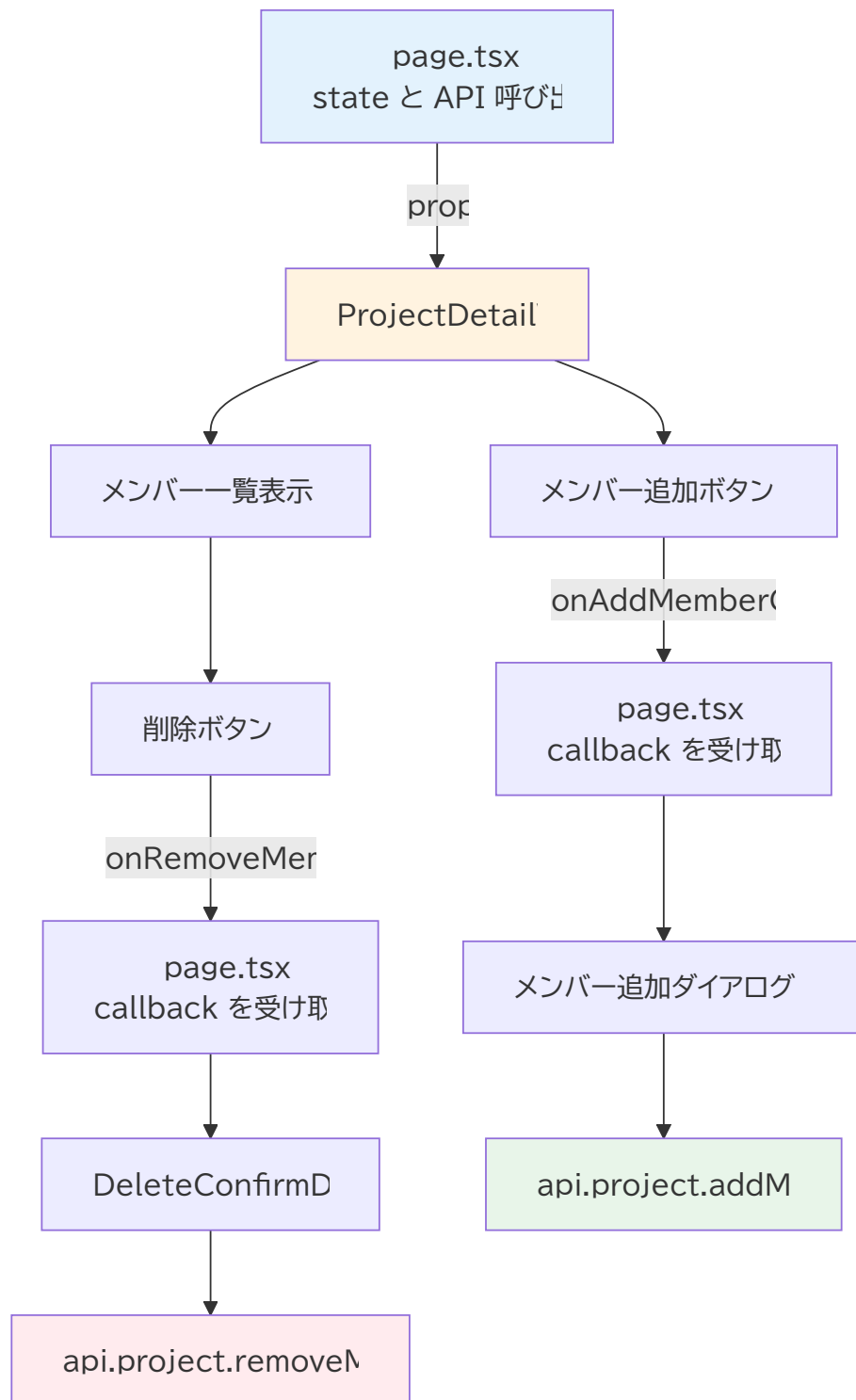
図 2: メンバー管理の構造
