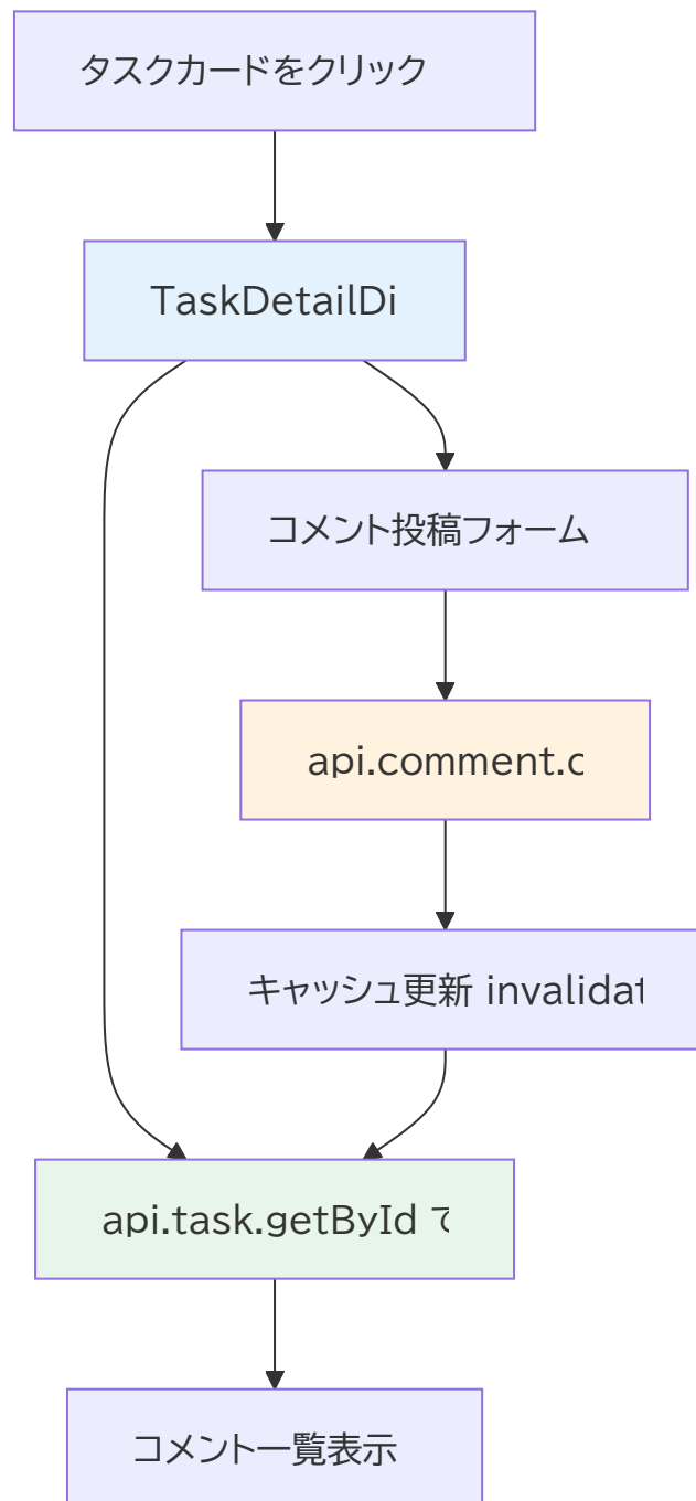
図 2: コメント機能の構成
