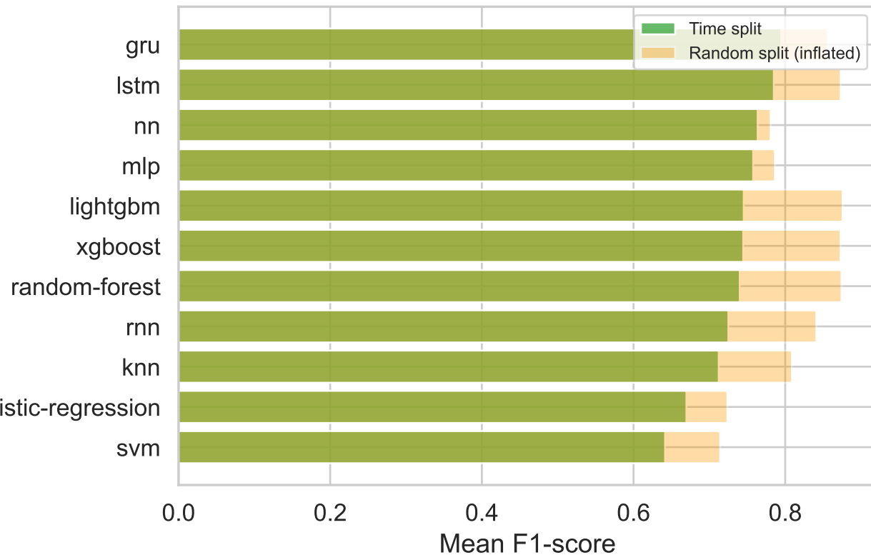
All Models: Time-split vs Random-split F1
