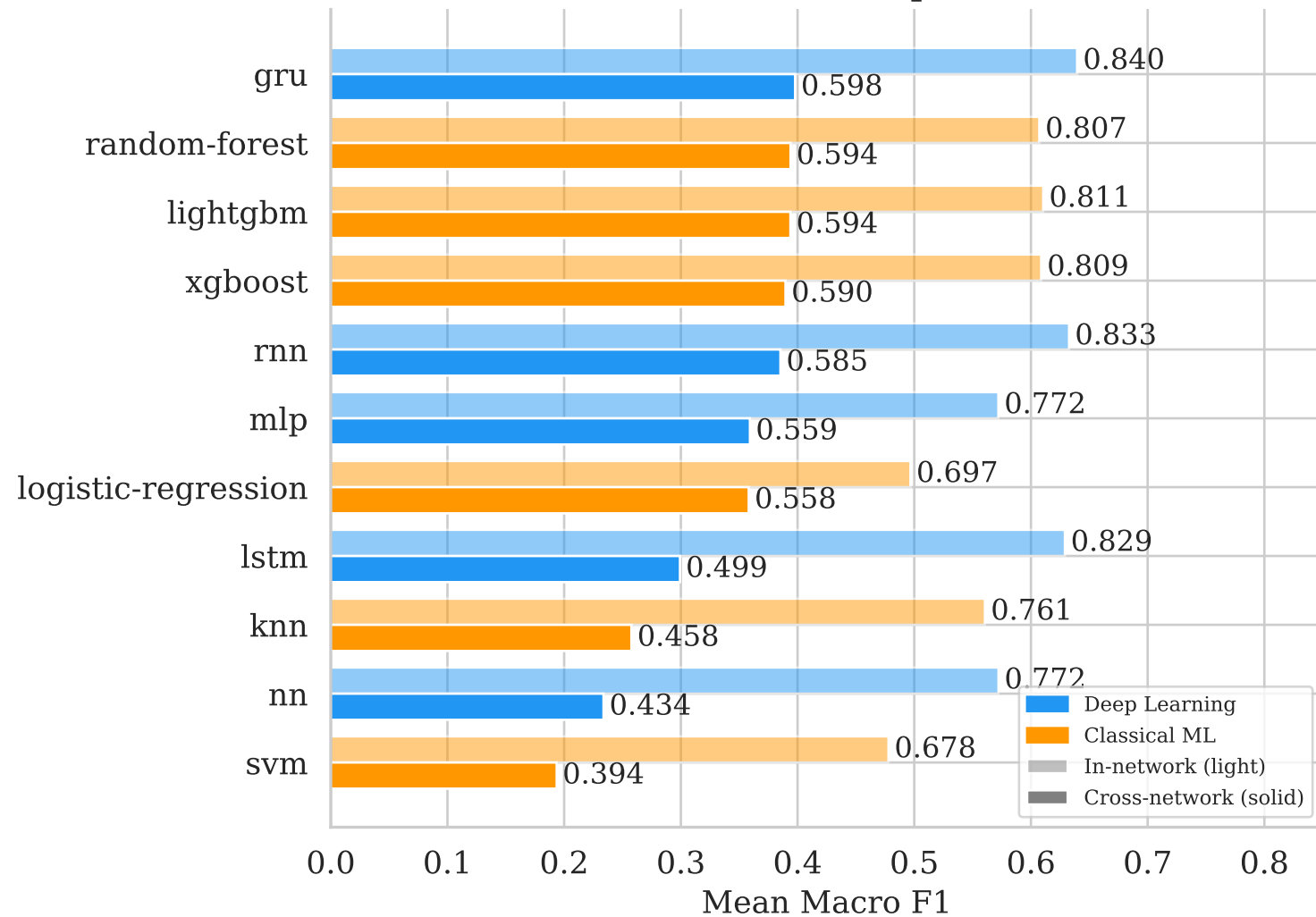
(a) Mean Macro F1 per model
