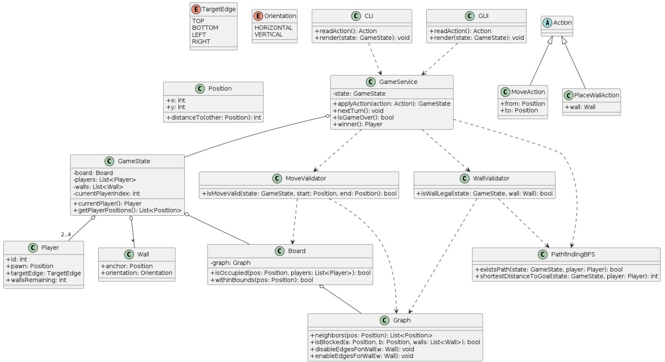
FIGURE 5 – Diagramme de classes UML du système Quoridor
