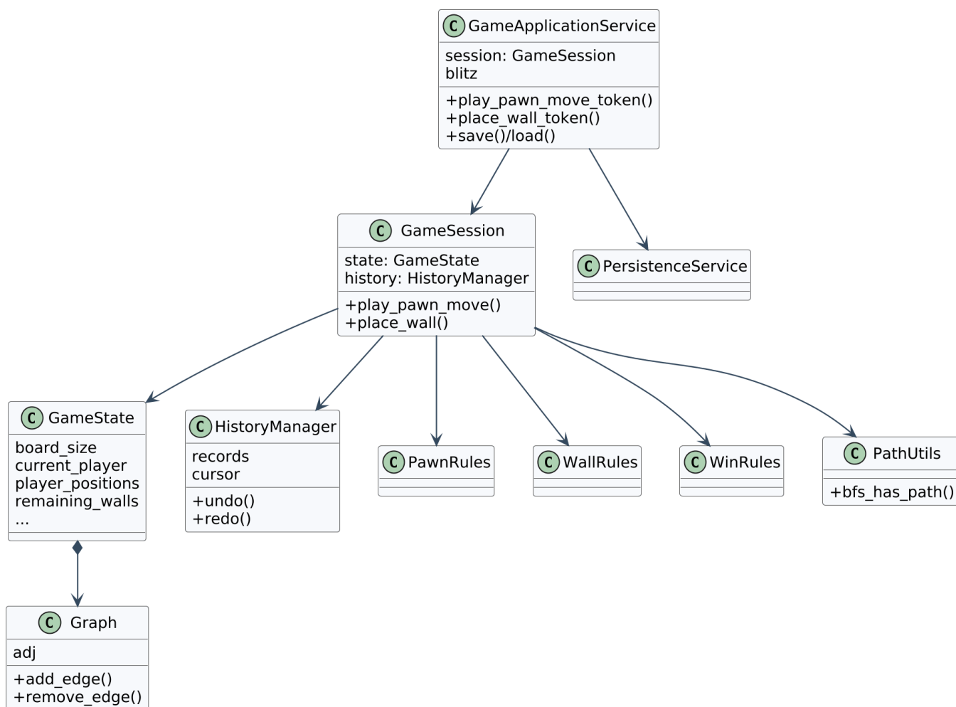
FIGURE 1 – Vue UML du noyau métier et de la couche applicative
