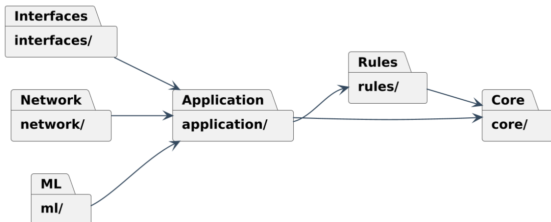
FIGURE 3 – Architecture modulaire de quoridor/ et dépendances principales
