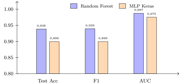
Figure 10 – Comparaison Random Forest / MLP sur le jeu de test
