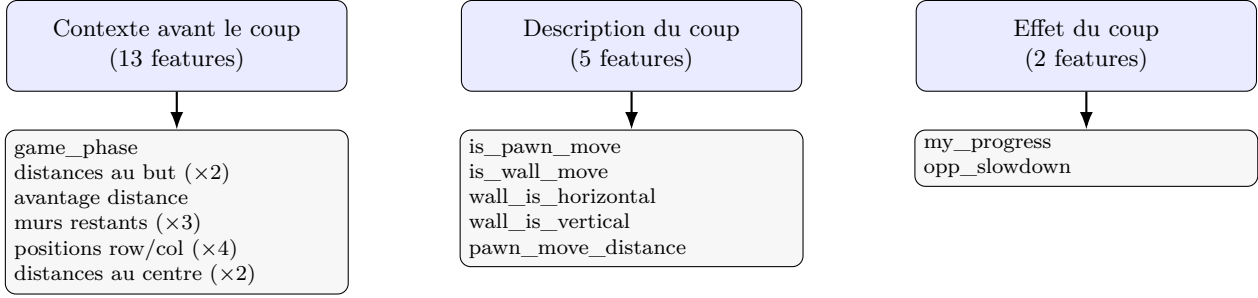
FIGURE 8 – Les 20 features utilisées pour la sélection ML
