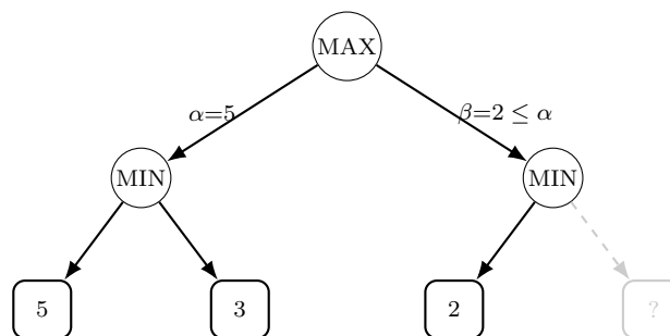
FIGURE 4 – Élagage alpha-beta : la branche droite est coupée car MIN a trouvé 2 alors que MAX dispose déjà d'une branche à 5.
