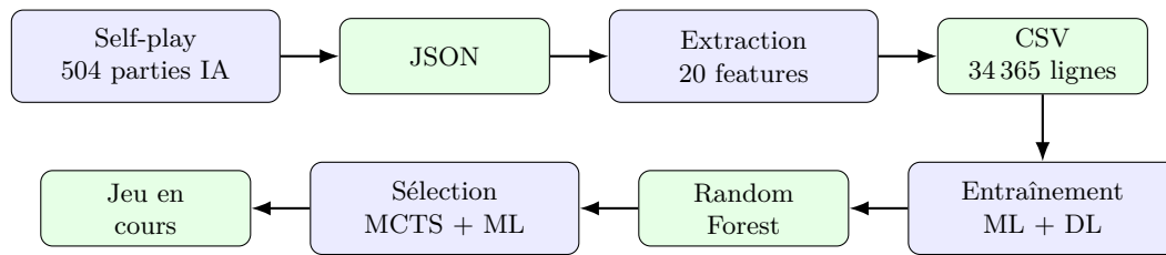
FIGURE 6 – Pipeline ML : génération, entraînement et intégration en jeu
