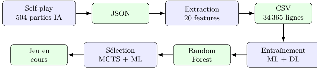
FIGURE 10 – Pipeline ML : génération, entraînement et intégration en jeu
