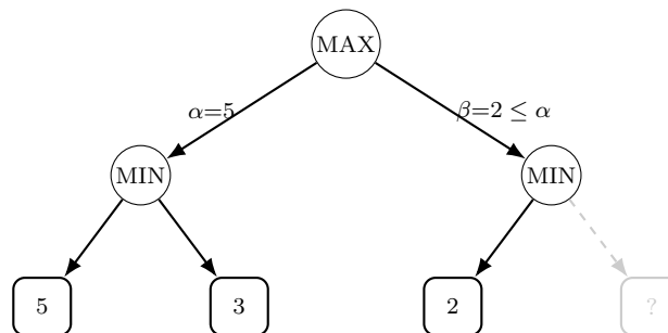
FIGURE 7 – Élagage alpha-beta : la branche droite est coupée car MIN a trouvé 2 alors que MAX dispose déjà d'une branche à 5.
