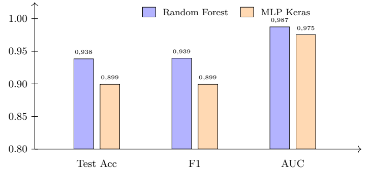
Figure 10 – Comparaison Random Forest / MLP sur le jeu de test
