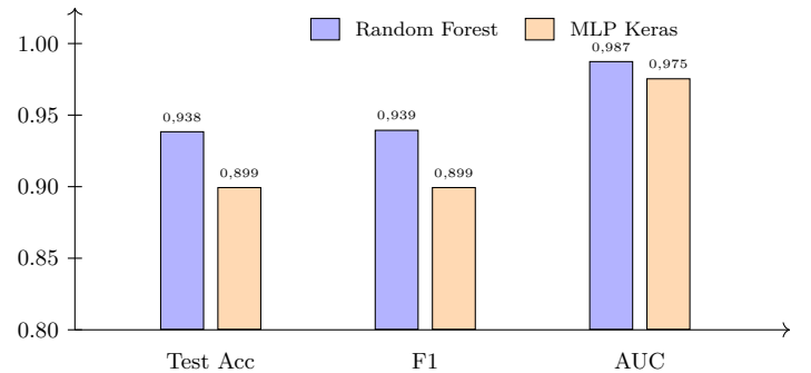
Figure 9 – Comparaison Random Forest / MLP sur le jeu de test
