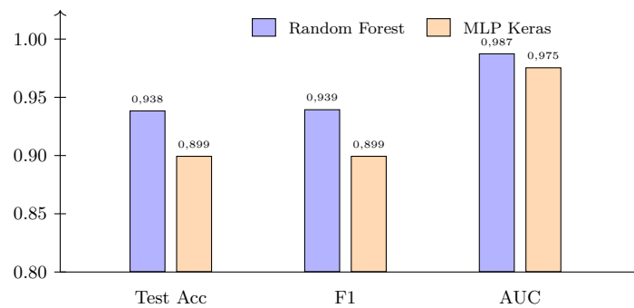
FIGURE 9 – Comparaison Random Forest / MLP sur le jeu de test
