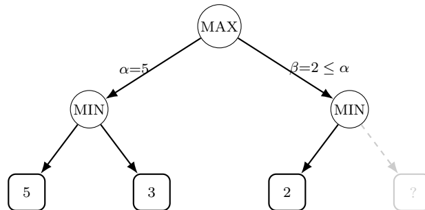
FIGURE 4 – Exemple d'élagage alpha-beta.
