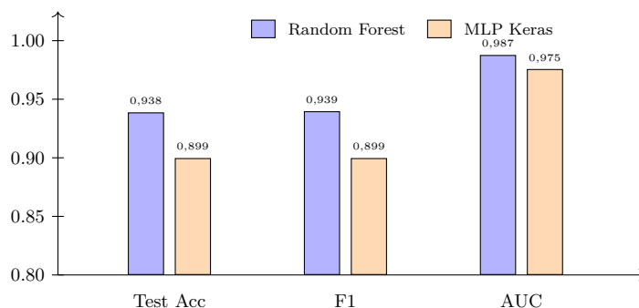
FIGURE 13 – Comparaison Random Forest / MLP sur le jeu de test
