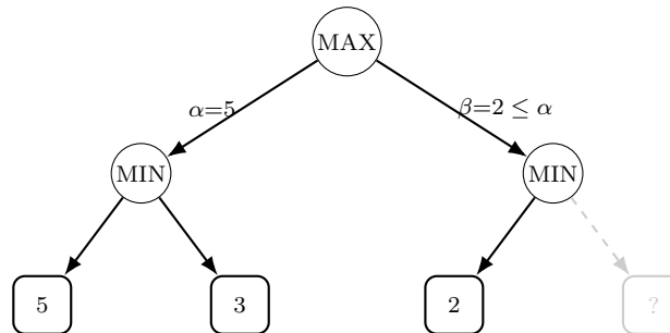
FIGURE 7 – Exemple d'élagage alpha-beta.
