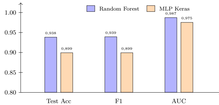
FIGURE 12 – Comparaison Random Forest / MLP sur le jeu de test
