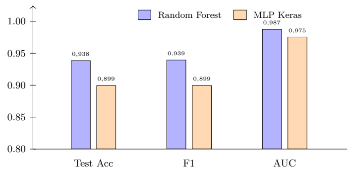
FIGURE 8 – Comparaison Random Forest / MLP sur le jeu de test
