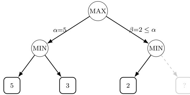
FIGURE 3 – Exemple d’élagage alpha-beta.
