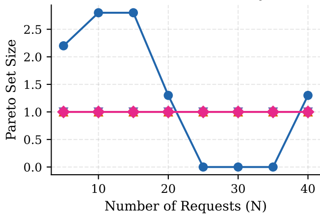
(d) Trade-off Diversity
