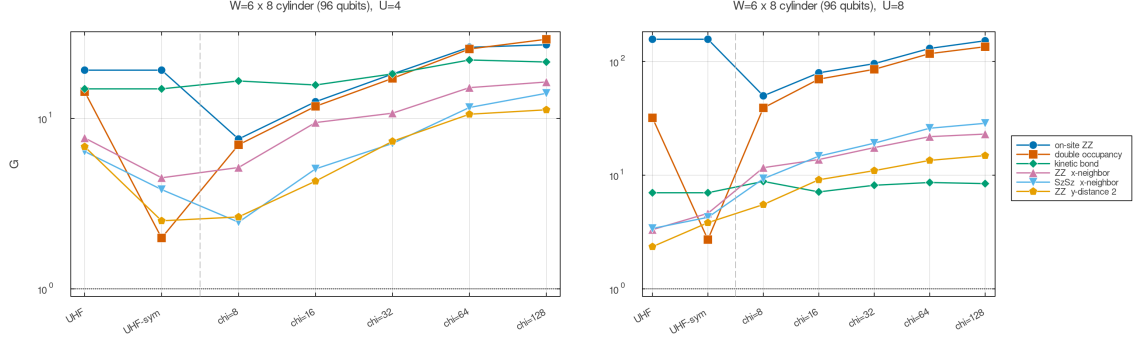
図 5: W = 6 シリンダー (96 量子ビット、クラスター計算)。安価 prior(UHF/UHF-sym) と切断 MPS の利得 (図は反復 30 回のモンテカルロの値で、本文の数値は厳密な式による)。 W = 4 に比べ MPS prior の立ち上がりが遅く、平均場の相対優位が拡大する。
