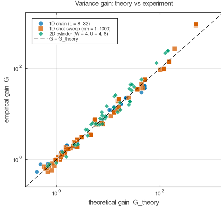
図 1: 利得法則のマスタープロット。1 次元鎖 ( L 掃引)、ショット配分掃引 ( n_m = 1-1000 )、2 次元シリンダー ( U = 4, 8 ) の全純 Pauli 列 (計 258 点) について、経験利得 G と理論値 (13) が対角線上に乗る (約 5 桁)。
