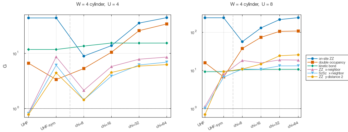
図 4: W = 4 シリンダーでの prior 比較 ( U = 4, 8 )。横軸左から UHF / UHF-sym / (縦破線) / 切断 MPS \chi = 8-64 。対称性回復でサイト間スピン相関 (桃・水色・橙) が MPS 系に並ぶ。
