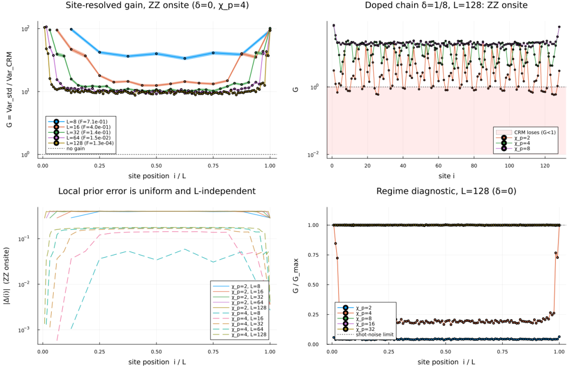
図 3: サイト分解した CRM 利得。(a) G(i) は L 非依存のバルク平坦部と端の増強を持つ。(b) ドープ系では粗い \text{prior}(\chi_p = 2) がサイトによって損をする。(c) 局所 prior 誤差 |\Delta(i)| はサイトにも L にもほとんど依存しない — 局所性の最も直接的な証拠。(d) G/G_{\max} による律速レジームの診断。
