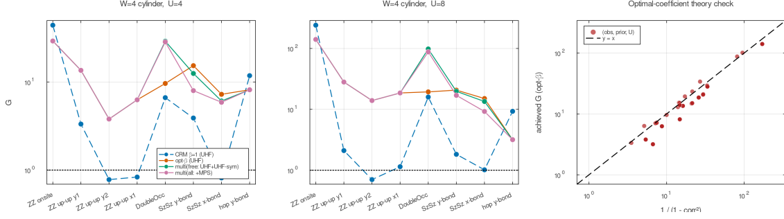
図 6: 最適係数 CRM と多 prior 回帰 ( W = 4, U = 4, 8 )。 \beta = 1 で G < 1 だった観測量が最適 \beta で全て G \geq 1 に修復 (右パネルで達成 G が理論 1/(1 - \text{corr}^2) に一致)。
