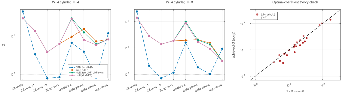
図 5: 最適係数 CRM と多 prior 回帰 ( W = 4, U = 4, 8 )。 \beta = 1 で G < 1 だった観測量が最適 \beta で全て G \geq 1 に修復 (右パネルで達成 G が理論 1/(1 - \text{corr}^2) に一致)。
