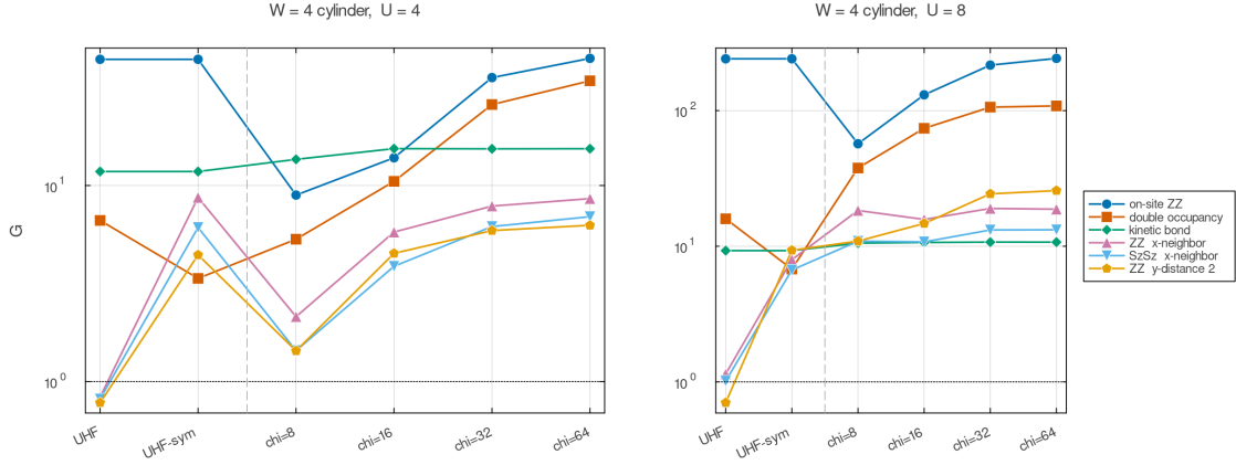
図 3: W = 4 シリンダーでの prior 比較 ( U = 4, 8 )。横軸左から UHF / UHF-sym / (縦破線) / 切断 MPS \chi = 8-64 。対称性回復でサイト間スピン相関 (桃・水色・橙) が MPS 系に並ぶ。
