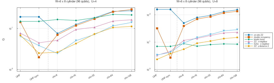
図 4: W = 6 シリンダー (96 量子ビット、クラスター計算)。安価 prior(UHF/UHF-sym) と切断 MPS の利得。 W = 4 に比べ MPS prior の立ち上がりが遅く、平均場の相対優位が拡大する。
