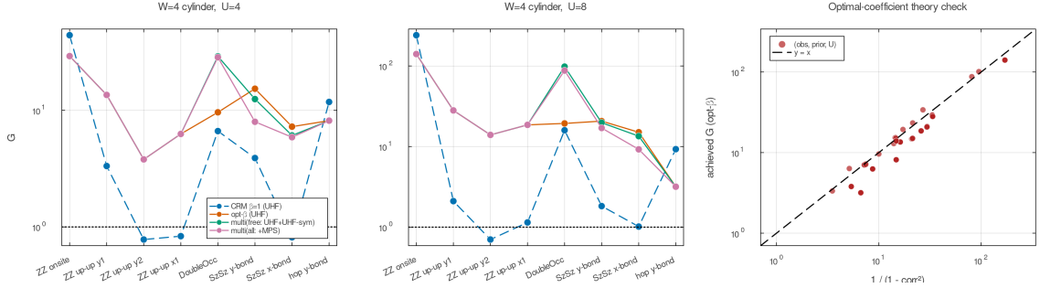
図 5: 最適係数 CRM と多 prior 回帰 ( W = 4, U = 4, 8 )。 \beta = 1 で G < 1 だった観測量が最適 \beta で全て G \geq 1 に修復 (右パネルで達成 G が理論 1/(1 - \text{corr}^2) に一致)。
