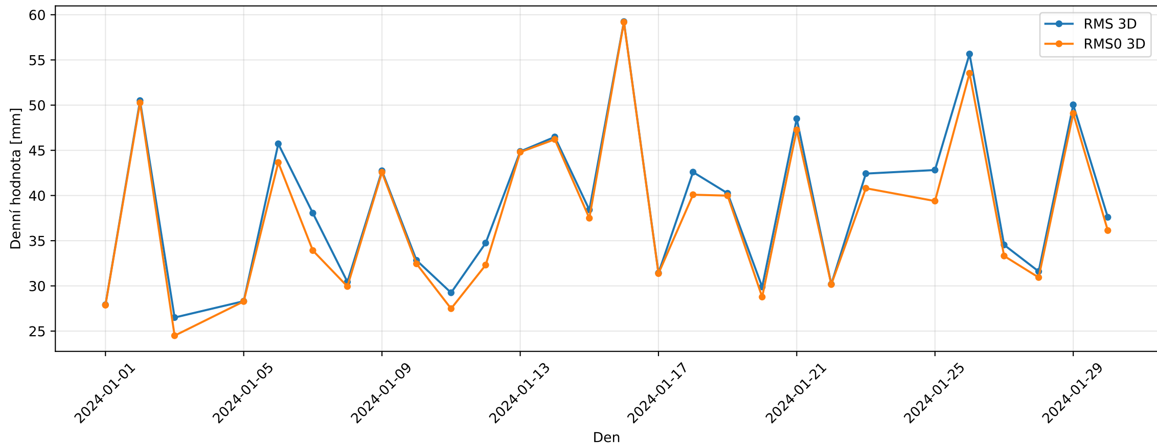
Porovnání RMS a RMS0 Bernese ZAZG — AS
