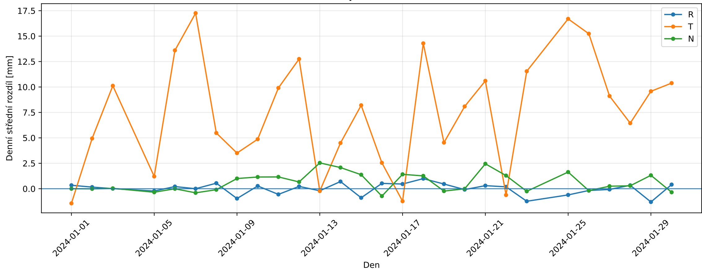
Denní střední rozdíly Bernese ZAZG v RTN — AS
