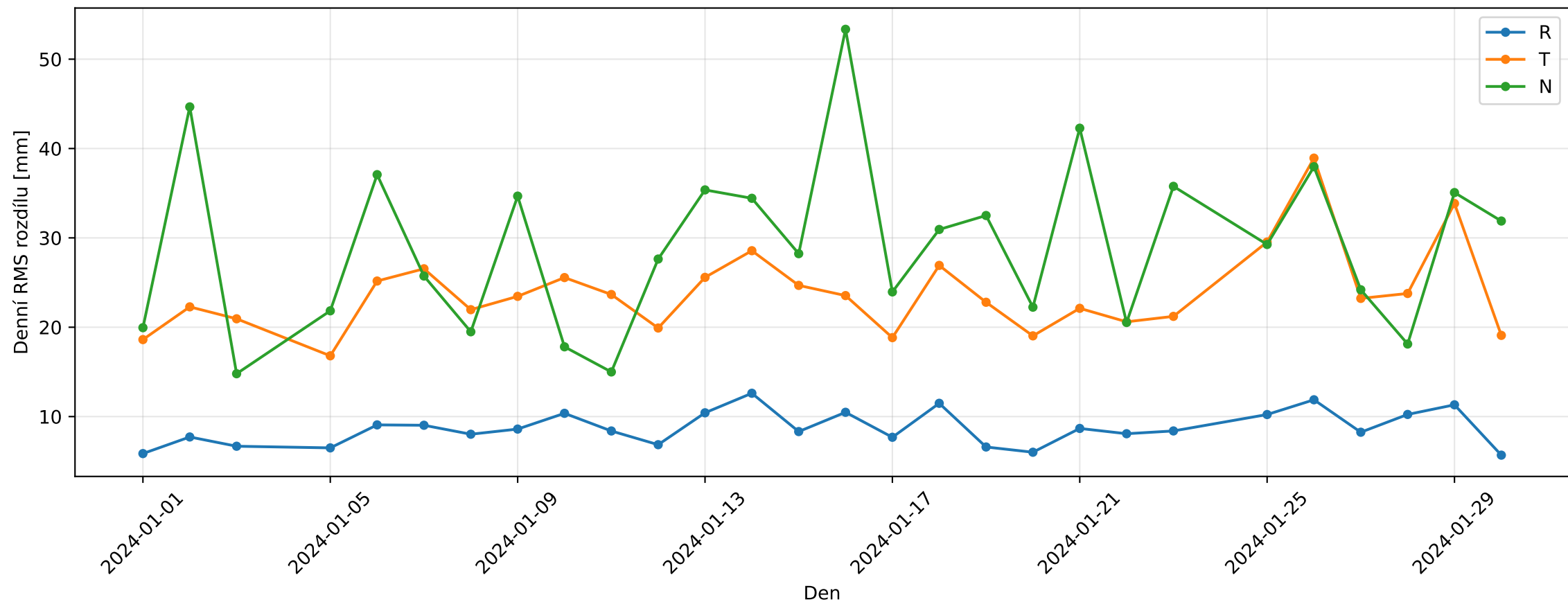
Denní RMS rozdílů Bernese ZAZG v RTN — AS
