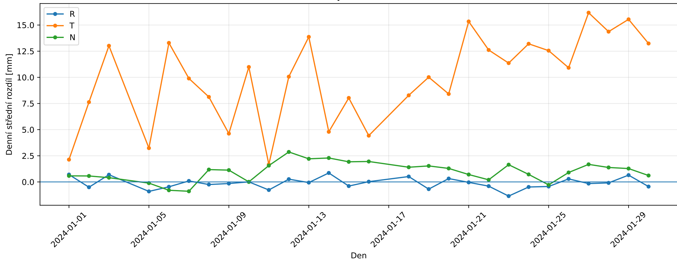
Denní střední rozdíly Bernese ZAZG v RTN — BS
