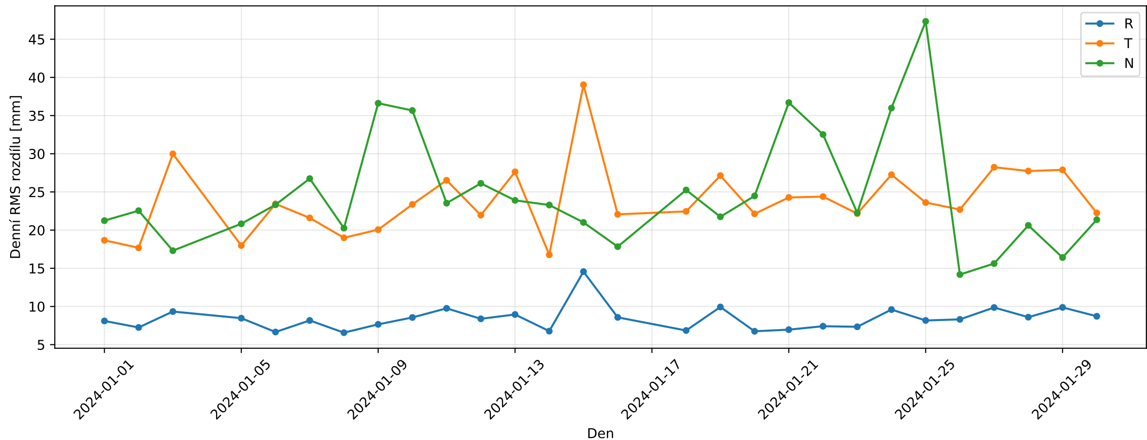
Denní RMS rozdílů Bernese ZAZG v RTN — BS
