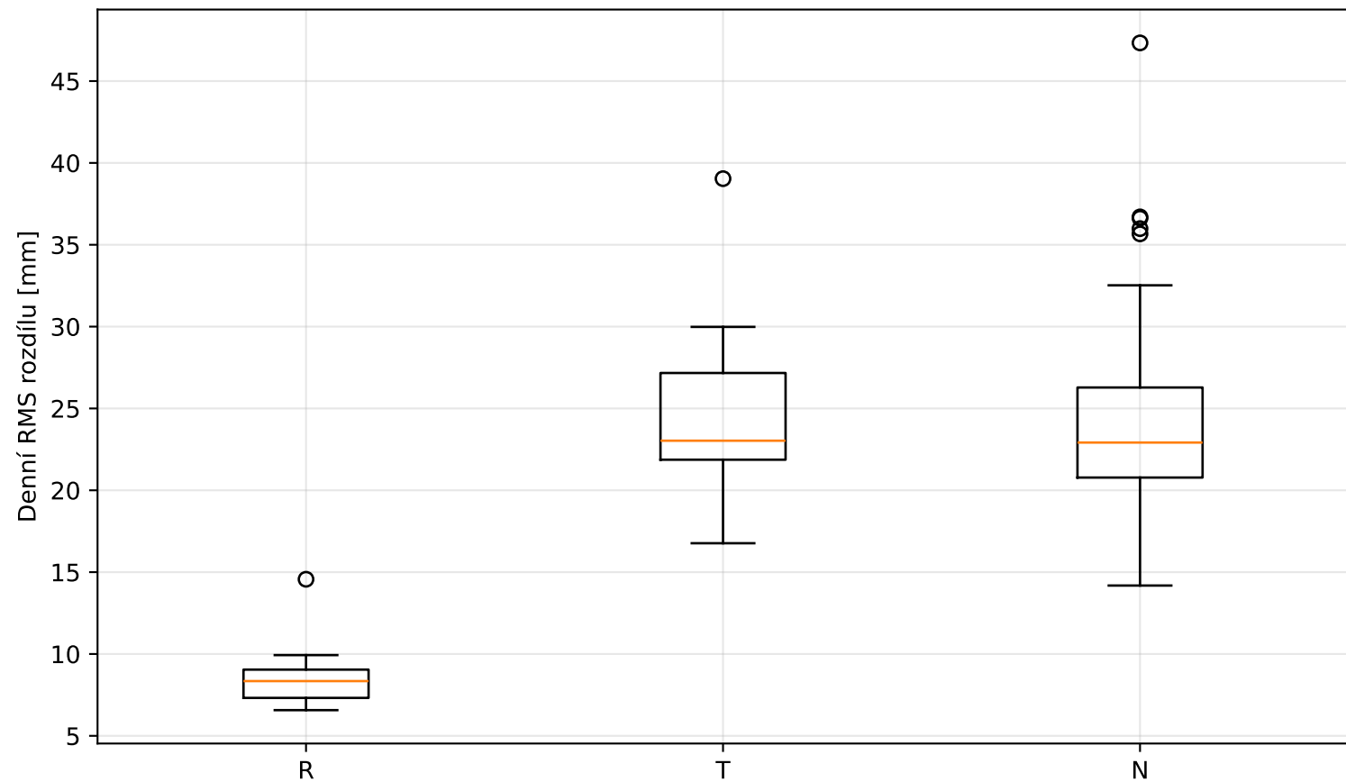
Rozdělení denních RMS rozdílů Bernese ZAZG — BS
