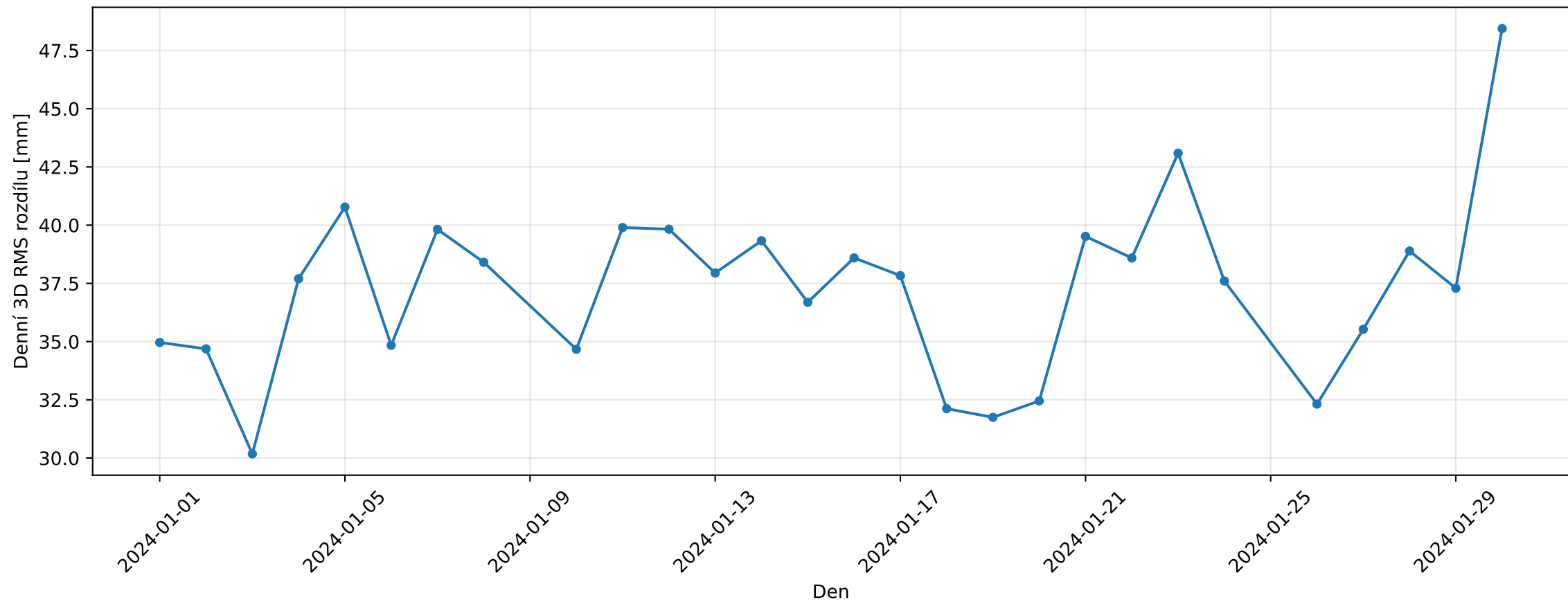
Denní 3D RMS rozdílů Bernese ZAZG — CR
