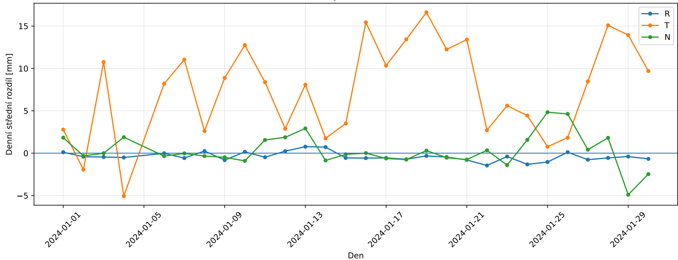
Denní střední rozdíly Bernese ZAZG v RTN — HC
