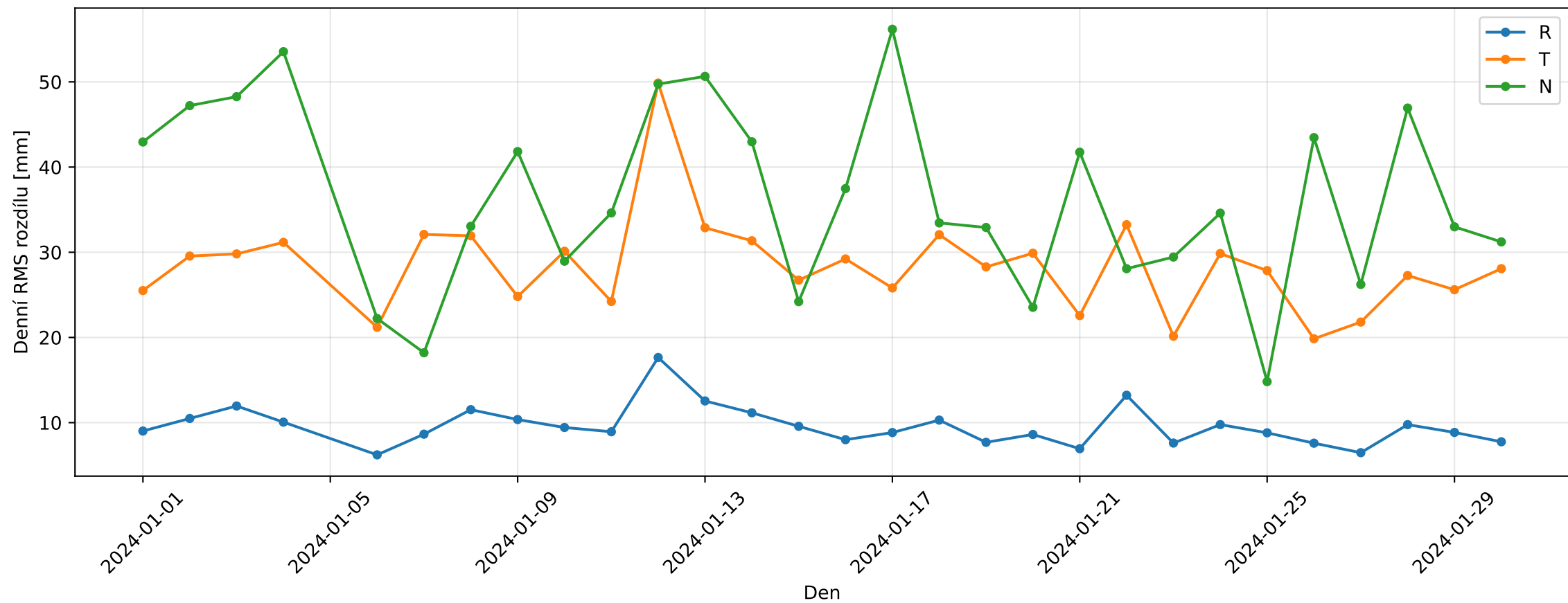
Denní RMS rozdílů Bernese ZAZG v RTN — HC
