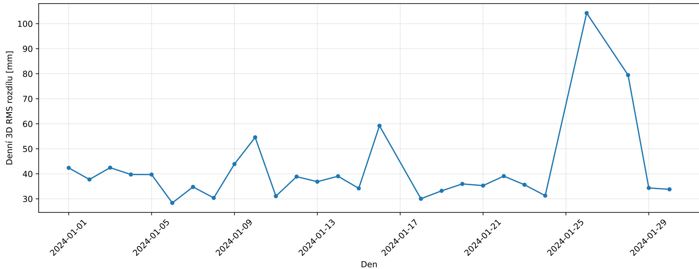
Denní 3D RMS rozdílů Bernese ZAZG — HD
