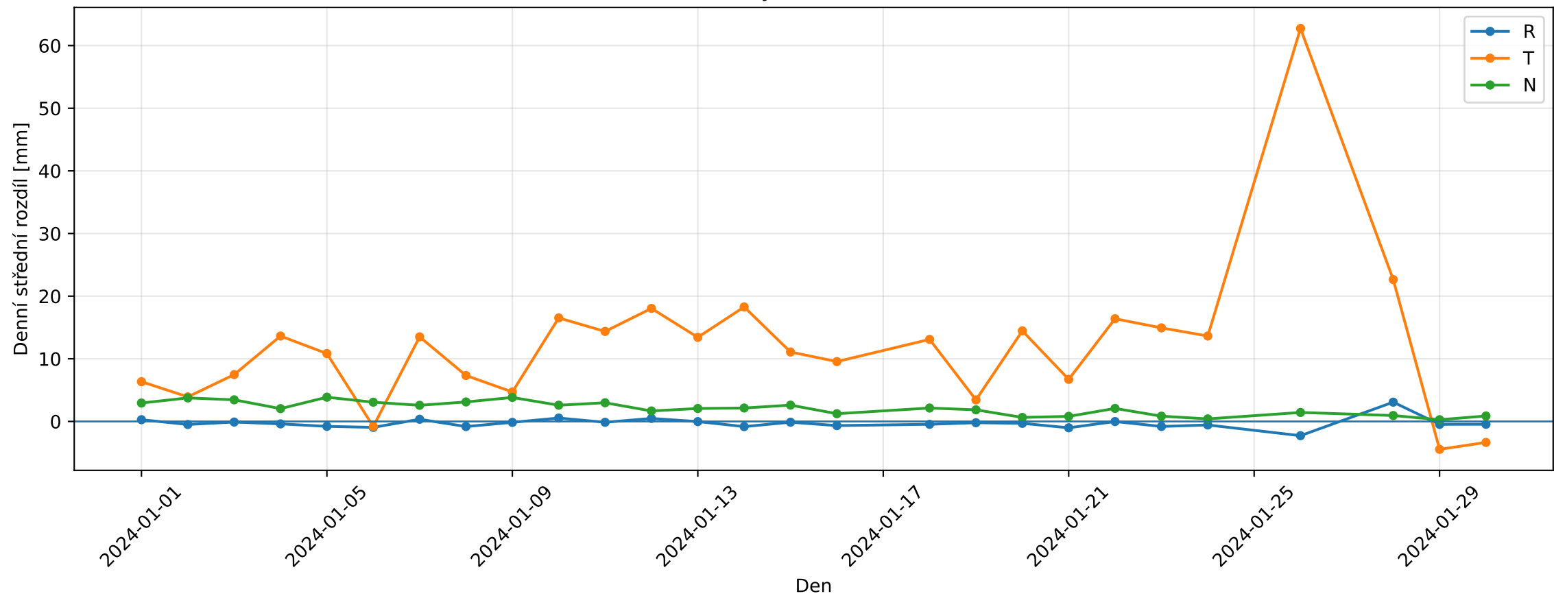
Denní střední rozdíly Bernese ZAZG v RTN — HD
