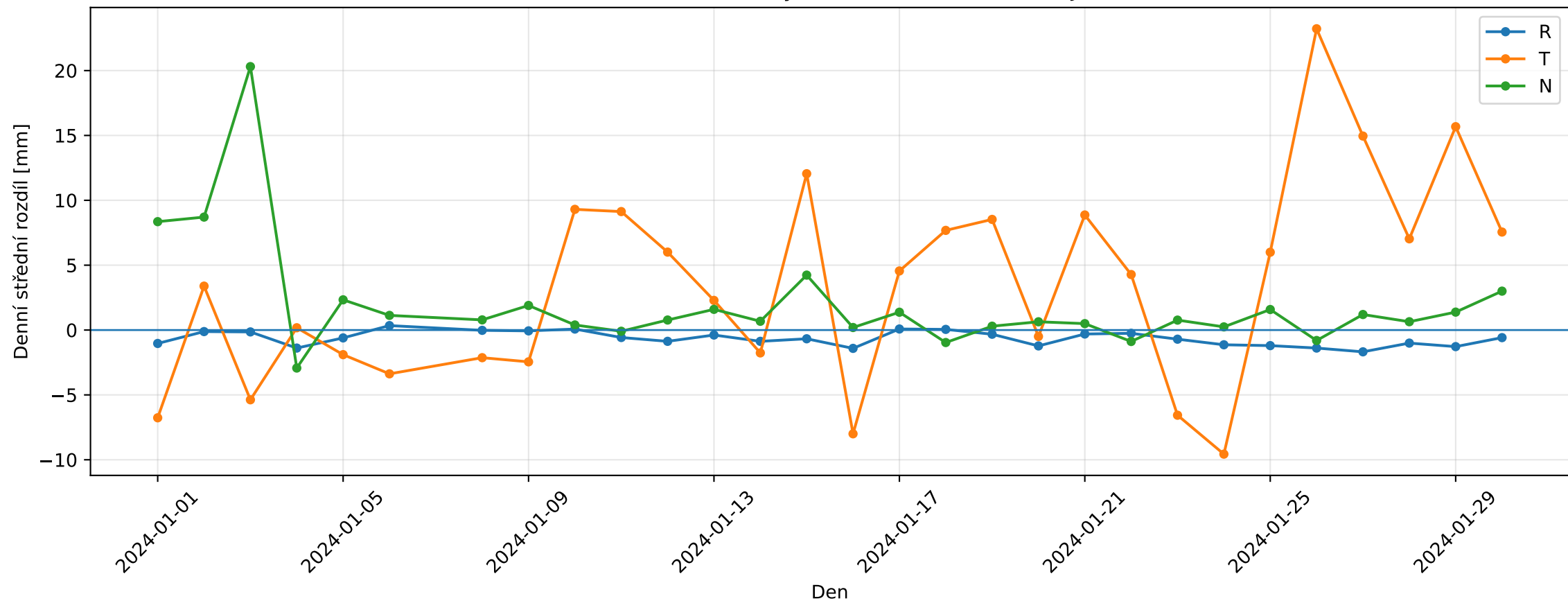
Denní střední rozdíly Bernese ZAZG v RTN — J3
