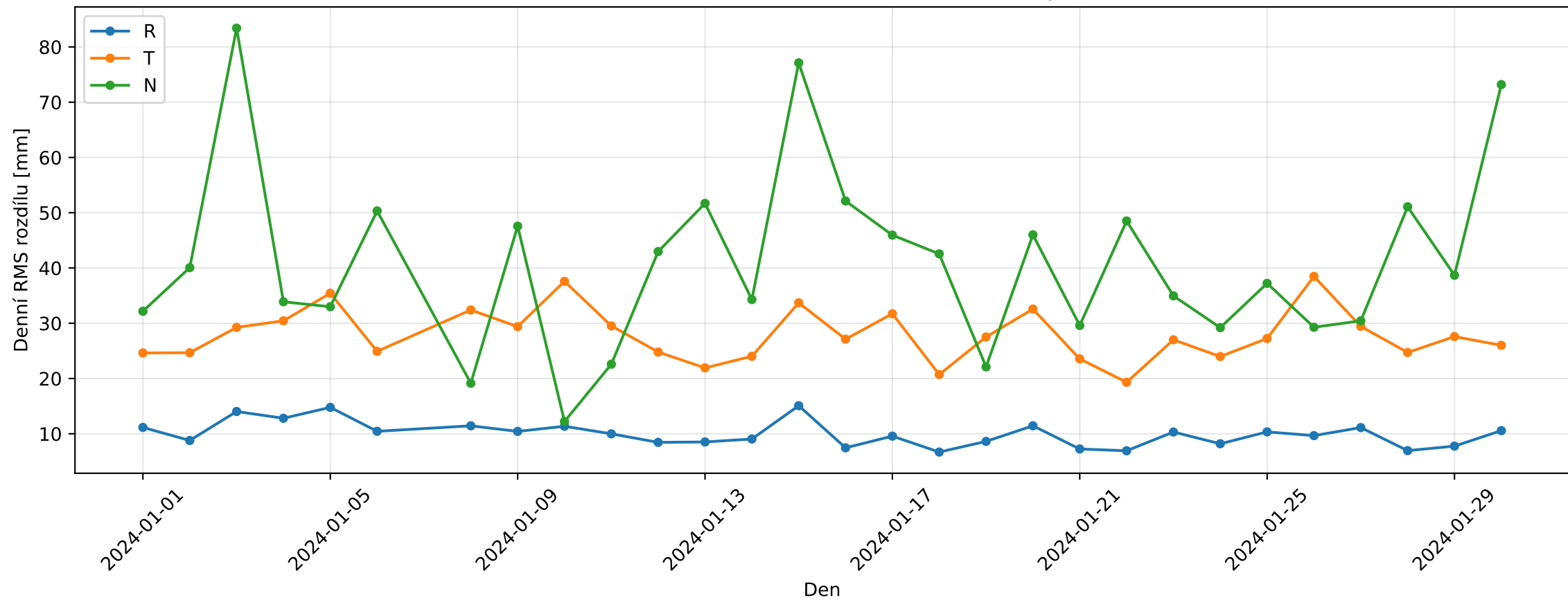
Denní RMS rozdílů Bernese ZAZG v RTN — J3
