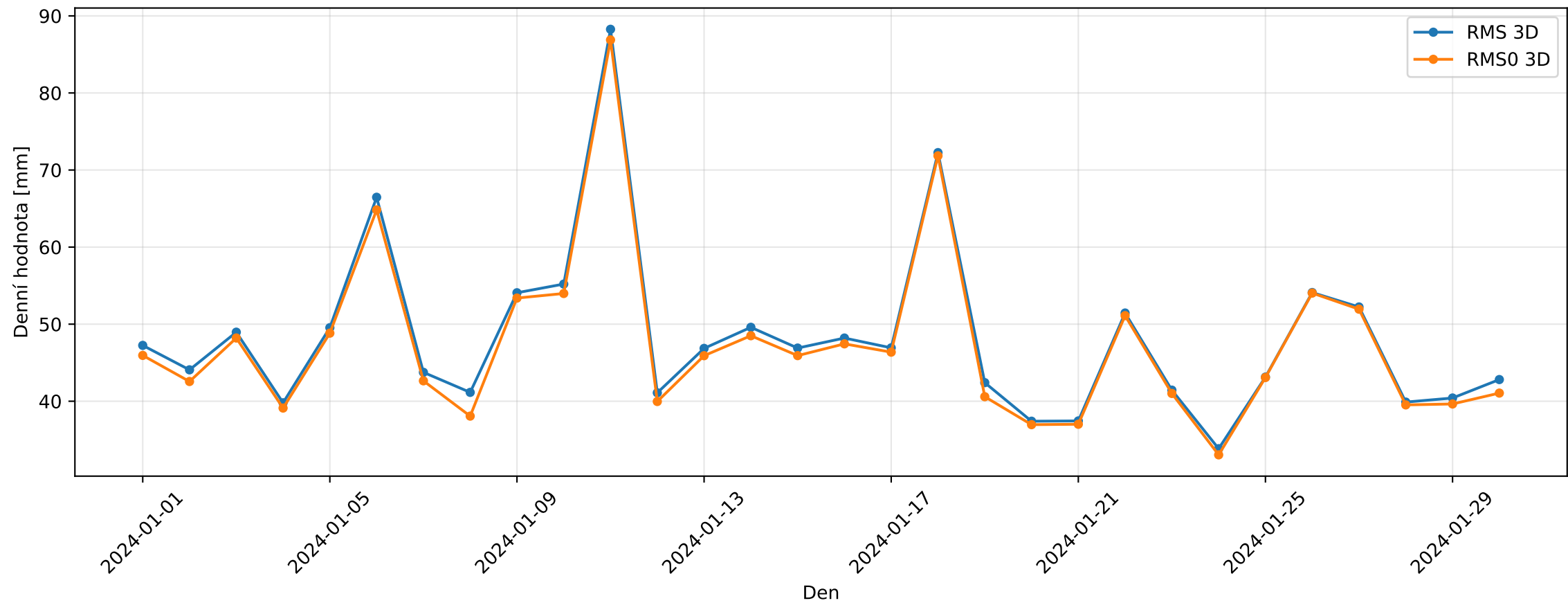
Porovnání RMS a RMS0 Bernese ZAZG — S6
