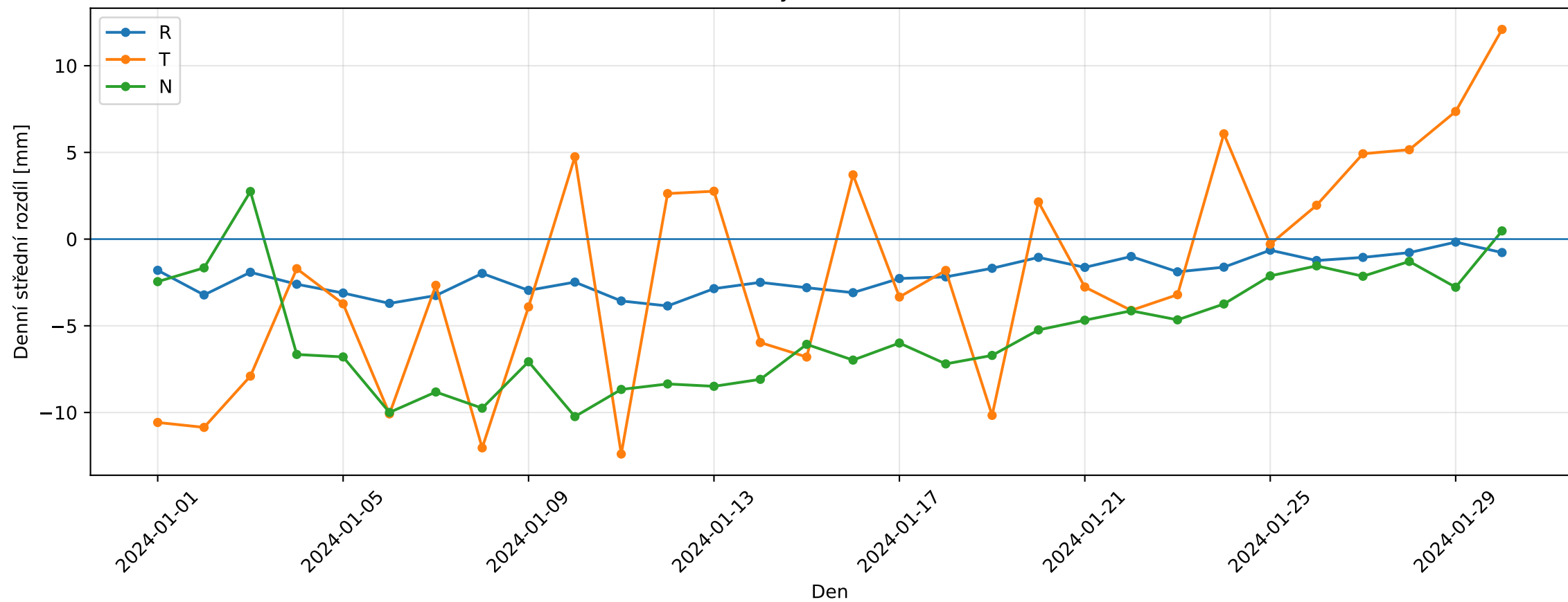
Denní střední rozdíly Bernese ZAZG v RTN — S6
