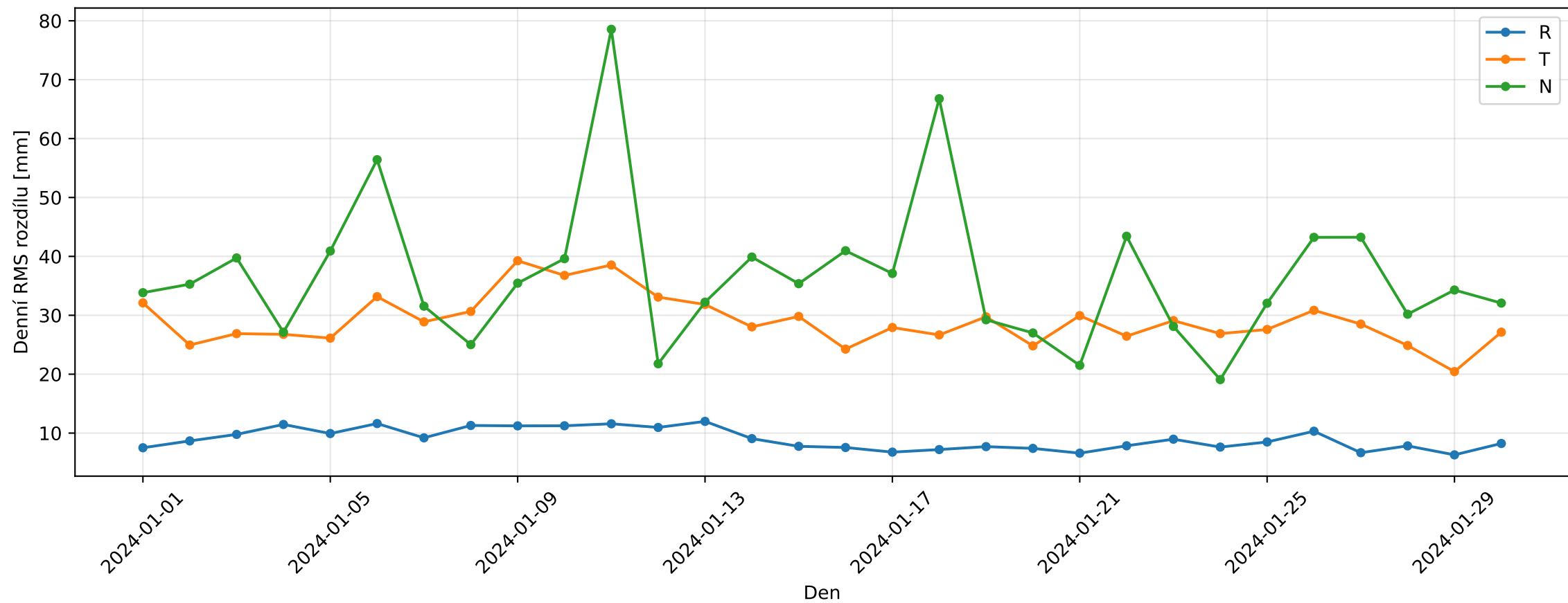
Denní RMS rozdílů Bernese ZAZG v RTN — S6
