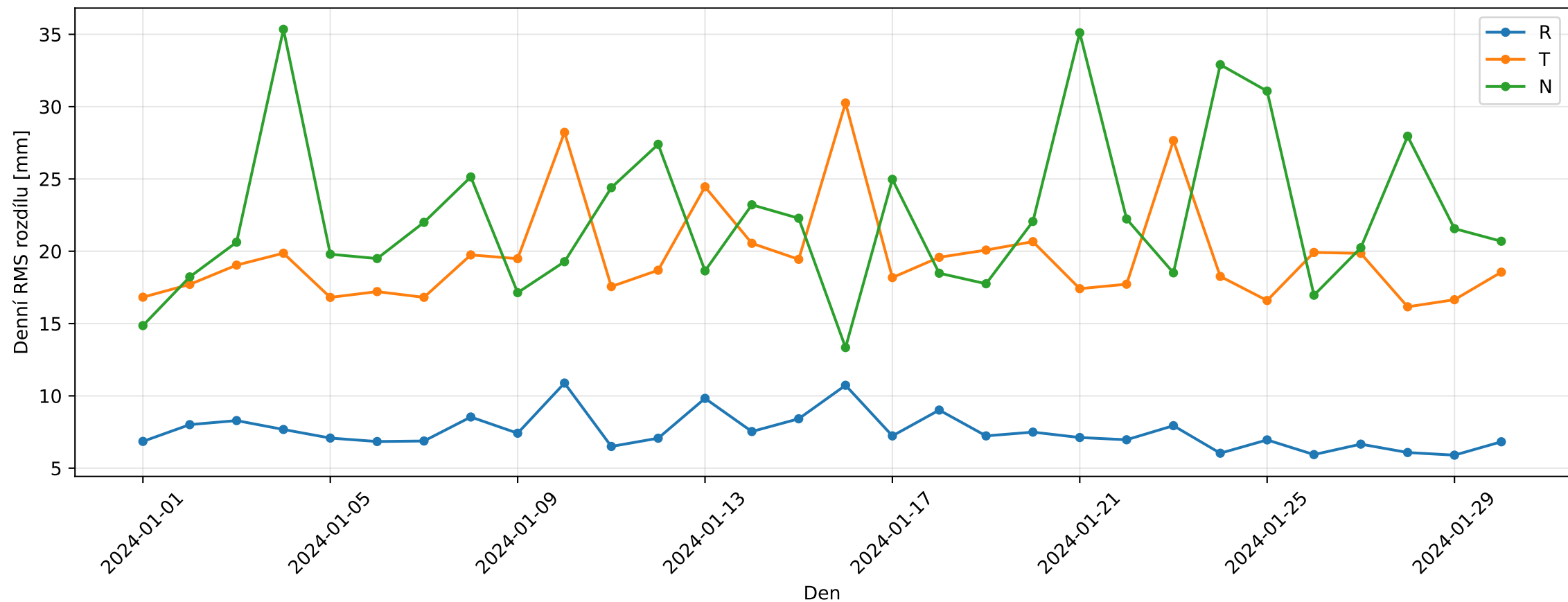
Denní RMS rozdílů Bernese ZAZG v RTN — SA
