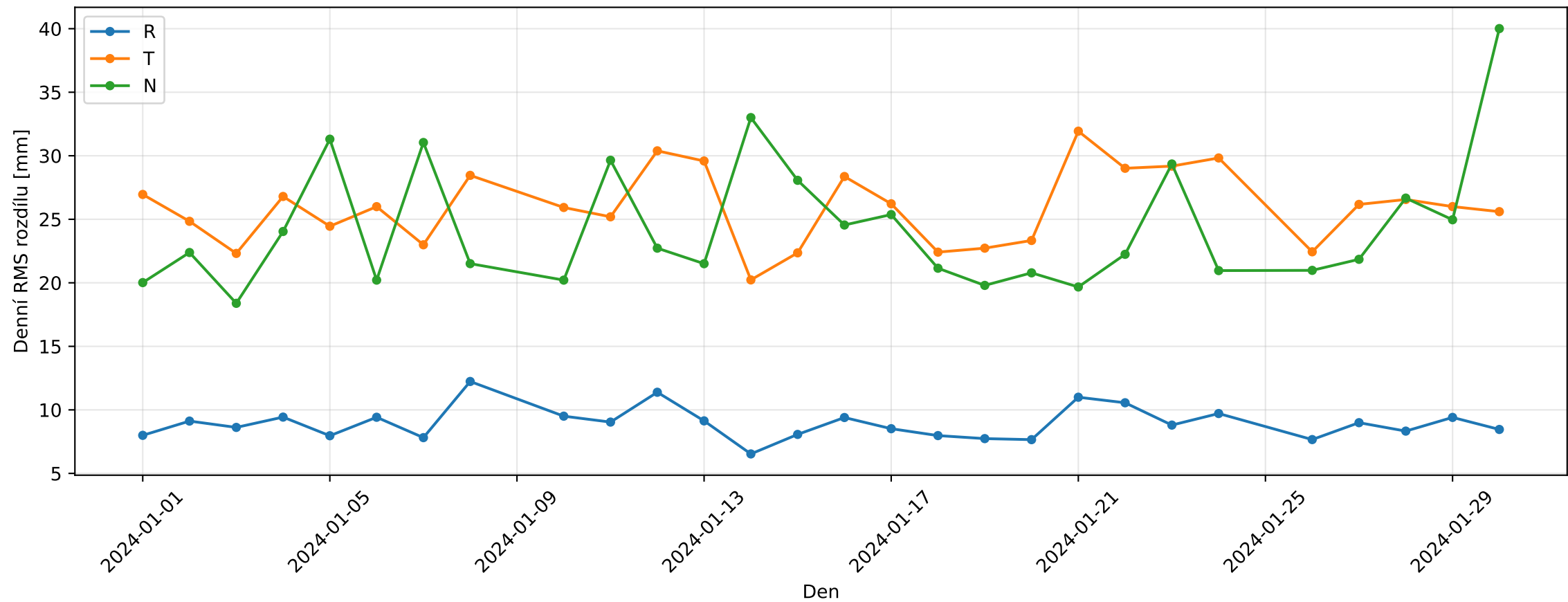
Denní RMS rozdílu mezi GOP a SSA v RTN — CS2
